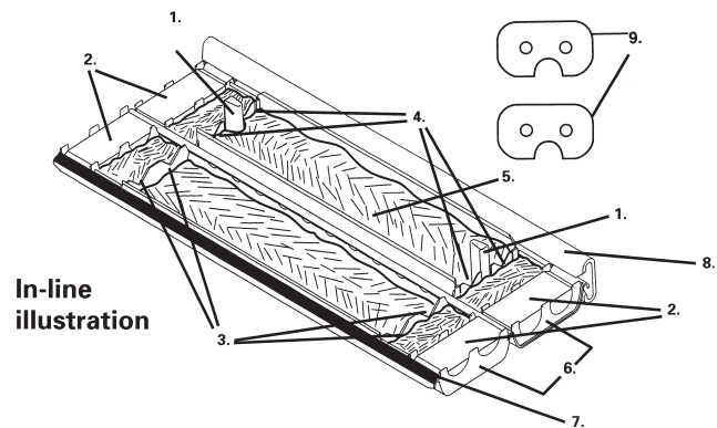
25-Pair Butt Version, Cat. No 8006318
